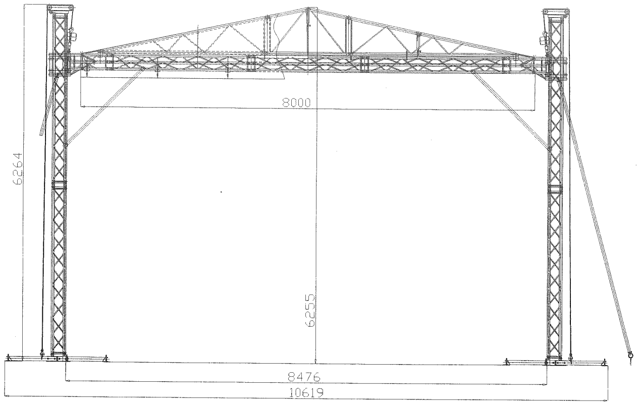
Rysunek 1. Widok zadaszania z przodu
